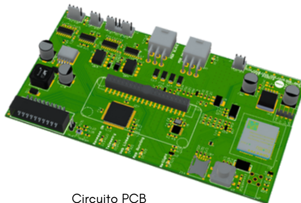
Circuito PCB
